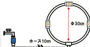
ミスト3個仕様 全長約10.3m
